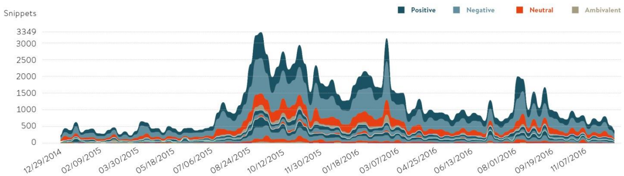
Abbildung: Sentiment-Verlauf 2014-2016
